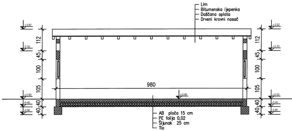
PRESJEK B-B
