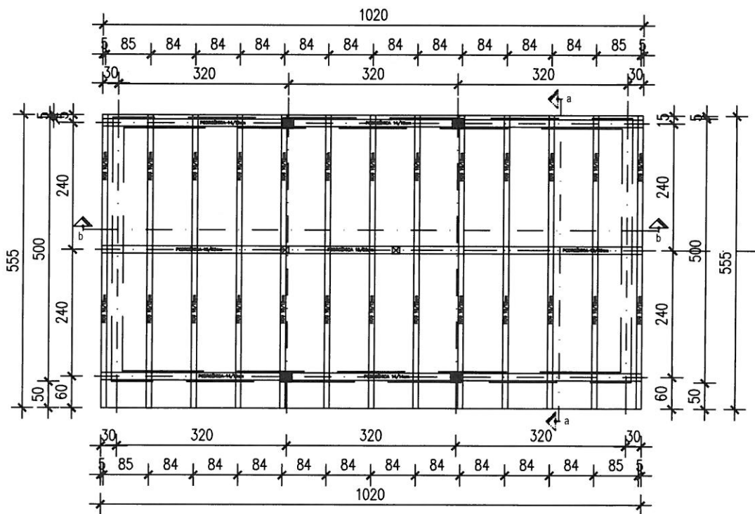
TLOCRT KROVIŠTA
