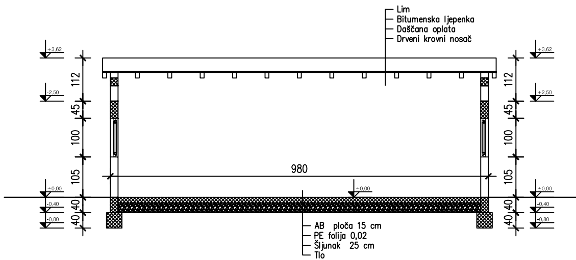
PRESJEK B-B
