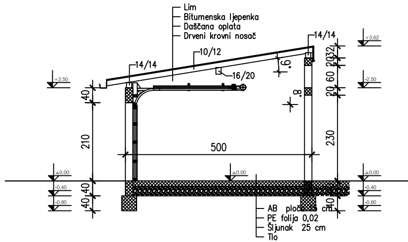
PRESJEK A-A
