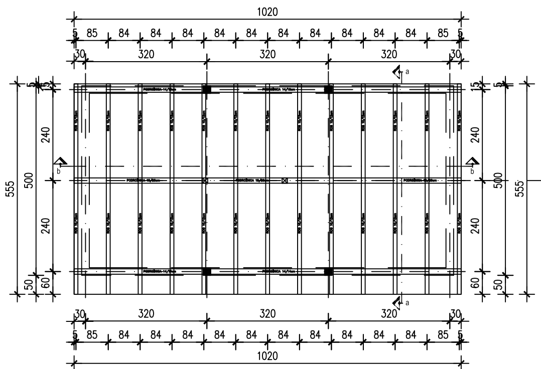
TLOCRT KROVIŠTA
