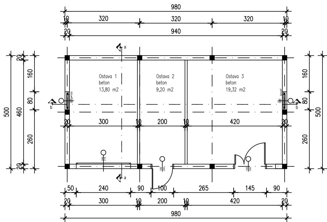
TLOCRT PRIZEMLJA
